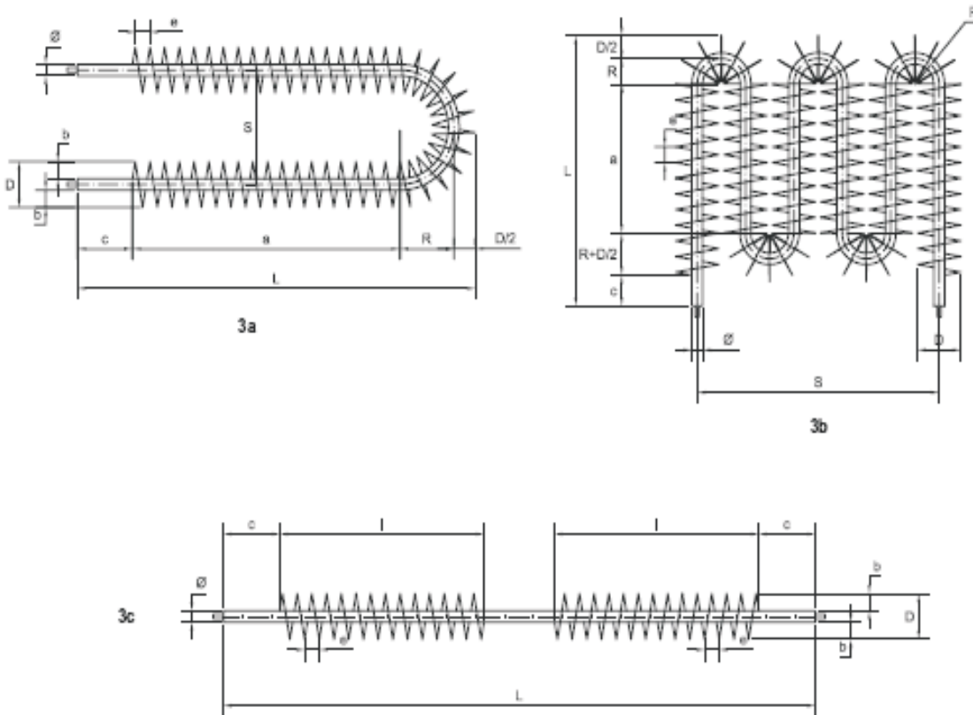
SLIKA 3: Tera cevni orebreni grejači
