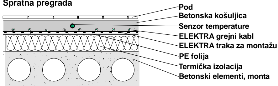
Slika 3d Presek poda sa instalacijom
