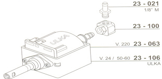
23 - 021 1/8" M
