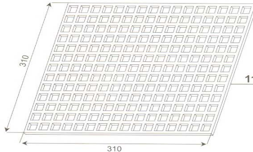
11 - 088
