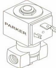
1/4 x 1/4 13 - 273 V. 220 / 50 - 60 14 - 209 V. 24 / 50 - 60
