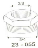
23 - 055
