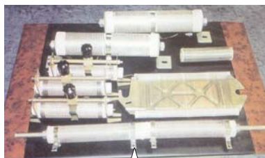
ОТПОРНИЦИ СО КЕРАМИЧКИ УЖЛЕБЕН НОСАЧ ФИКСНИ И РЕГУЛАЦИОНИ
