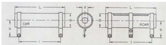
СЛ.1 - ИЗГЛЕД НА ЖИЧАН ОТПОРНИК СО ЦЕМЕНТЕН ПРЕМАЗ (ЦНПР)
