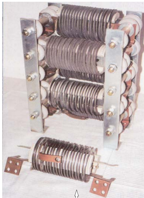
ОТПОРНИЦИ А.РП - ЛОКОМОТИВА
