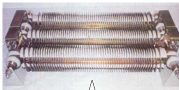
Сет отпорници за динамички кочници од електромоторен воз 412/416.
